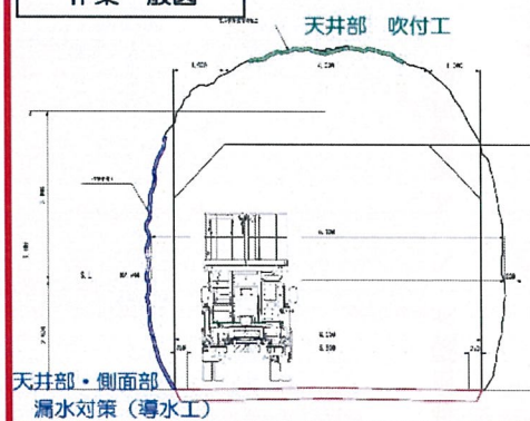
作業一般図
